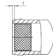
DETTAGLIO "A" POSIZIONE FILTRO SCALA 2:1
