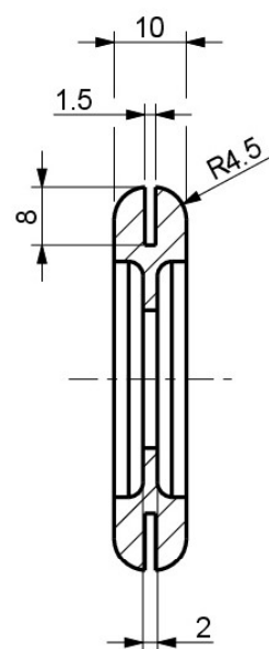
SEZIONE A-A
